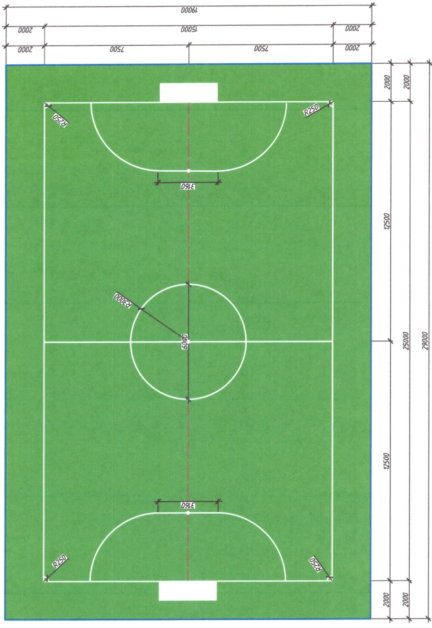
Разметка спортивной площадки 15,0 x 25,0 м
